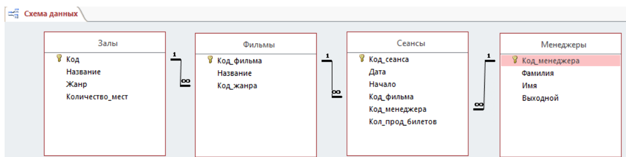
Рис. 1 Схема данных базы
